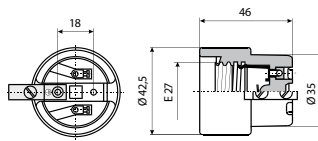
Porculansko grlo E 27 sa nosačem S
