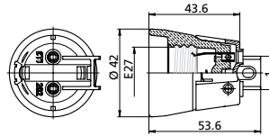
Porculansko grlo E 27-202
