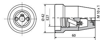
Porculansko grlo E 27 sa porc. poklopcem
