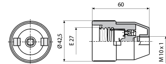
Porculansko grlo E 27 sa poklopcem P
