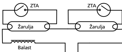
SERIJA 220-240 V~
