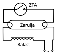
JEDNOSTRUKI 110-130 V~
