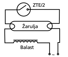
JEDNOSTRUKI 220-240 V~
