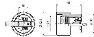
Porculansko grlo E 27 sa nosačem L
